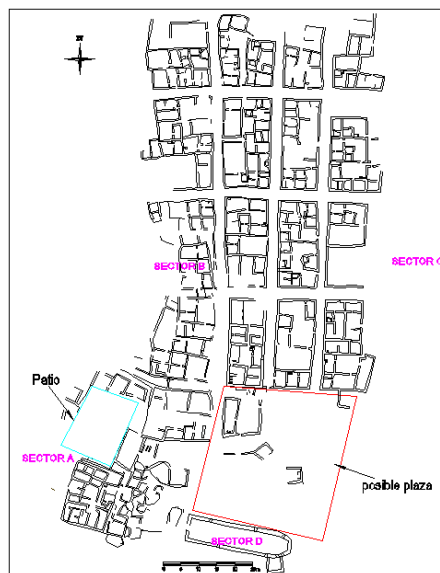
Figura 2: Plano donde se indica la plaza inca propuesta por algunos autores (derecha) y el espacio abierto adicional (izquierda) que proponemos
